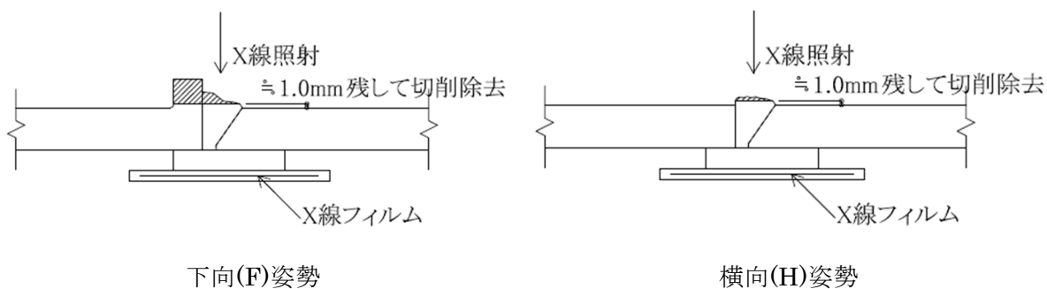
図10 X線撮影要領
