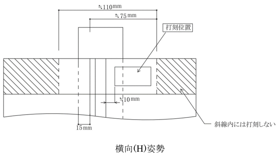
図4 マクロ試験体の刻印要領
