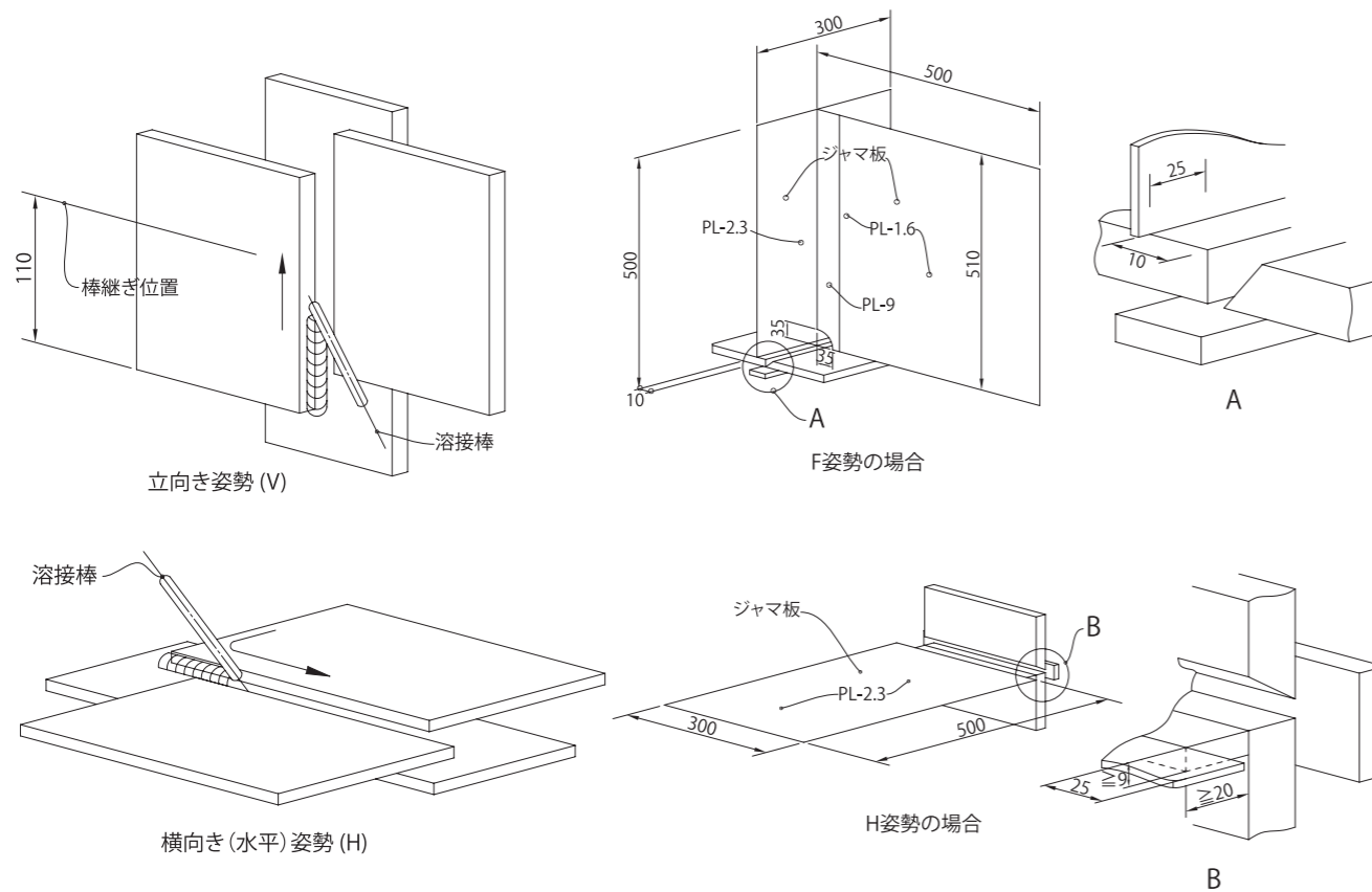
図3-3 溶接作業(すみ肉溶接の場合)
