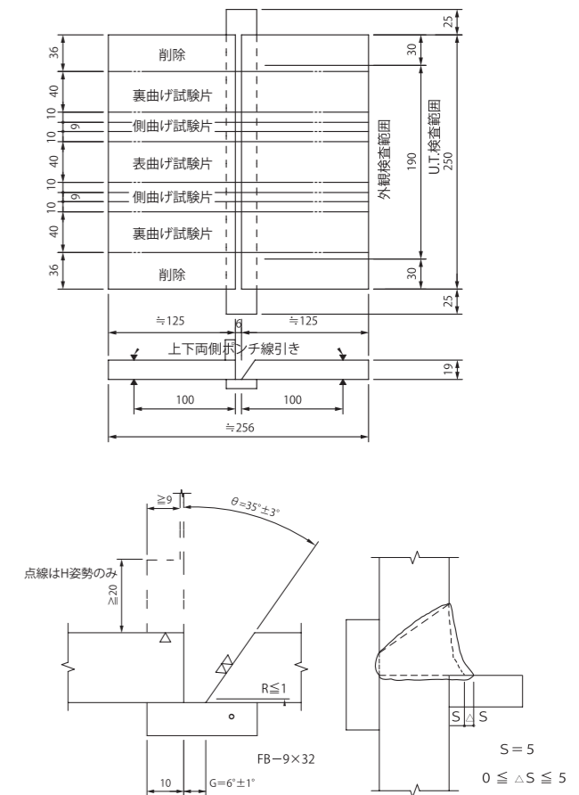
図3-2 試験材の形状 (2) 突合せ溶接
