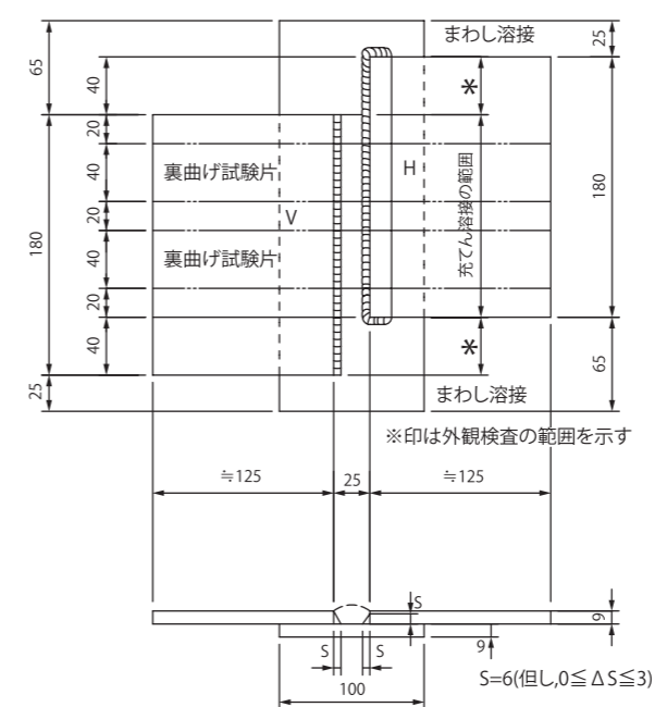
図3-1 試験材の形状 (1) すみ肉溶接
