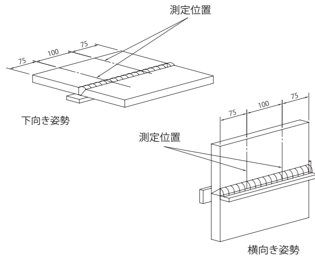
付図-2 突合せ溶接部の余盛及び脚長測定位置
