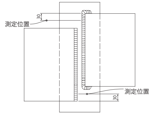
付図-1 すみ肉溶接部の脚長測定位置
