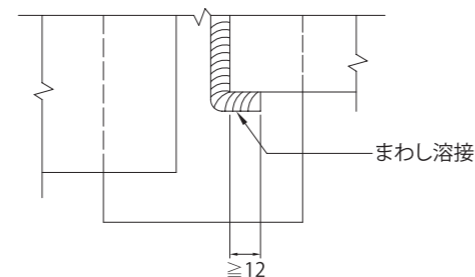
付図-4 十分なまわし溶接
